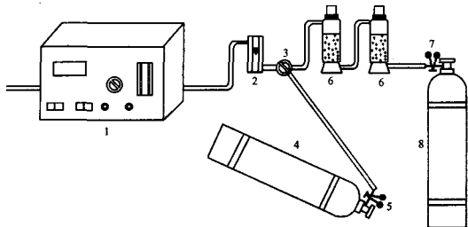
1—数字式微量水分仪；2—微量气体流量计；3—四通阀；4—六氟化硫气瓶； 5—氮气减压表；6—干燥塔；7—氮气减压表；8—氮气瓶
