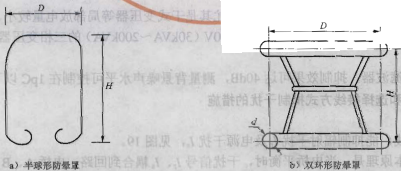
图 22 无晕环（球）结构图
