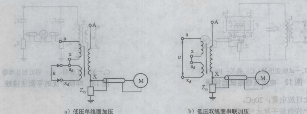
图9 电磁式电压互感器试验接线
