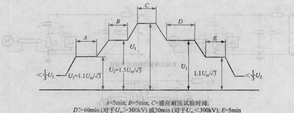
图5 变压器局部放电试验的加压时间及步骤
