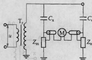
C_x —被试互感器； C_c —邻近互感器 图 13 抑制干扰的平衡法接线
