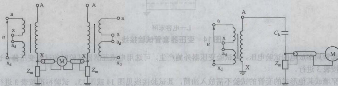
图10 抑制干扰的对称法接线
