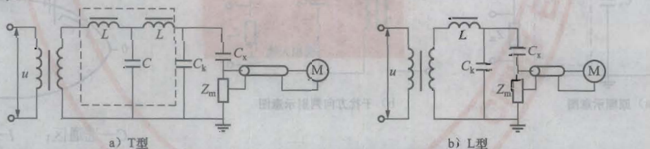
图 17 高压滤波器的接线图
