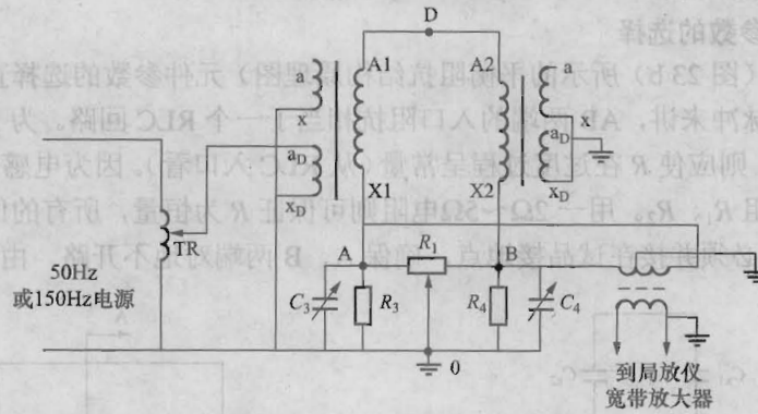
a) 电容式试品 (TA) 试验接线图
