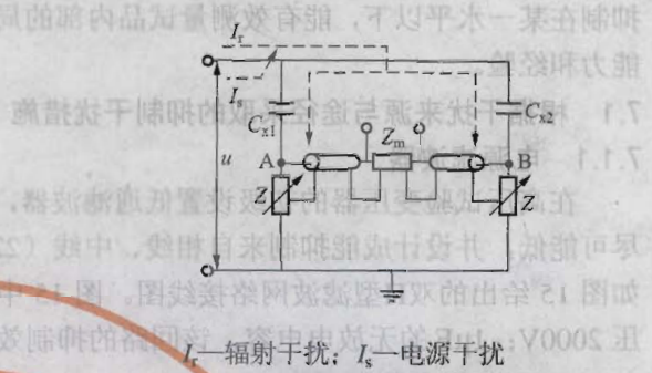
图 19 平衡法接线原理
