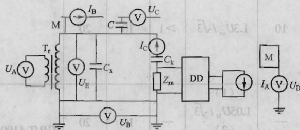
图 A.1 干扰及其进入试验回路的途径 Tr—试验变压器；Cx—被试品；Ck—耦合电容器；Zm—测量阻抗；DD—检测仪； M—邻近试验回路的金属物件；UA—电源干扰；UB—接地干扰；UC—经试验回路杂散电容 C 耦合产生的干扰；UD—悬浮电位放电产生的干扰；UE—高压各端部电晕放电的干扰；IA—试验变压器的放电干扰；IB—经试验回路杂散电感 M 耦合产生的辐射干扰；IC—耦合电容器放电的干扰
