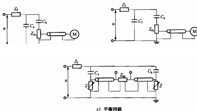
图 1 局部放电测量的基本回路
