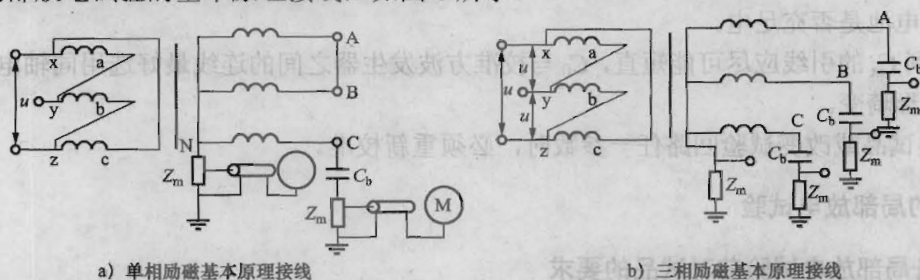
a) 单相励磁基本原理接线
